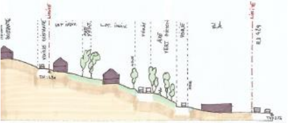
Coupe C
